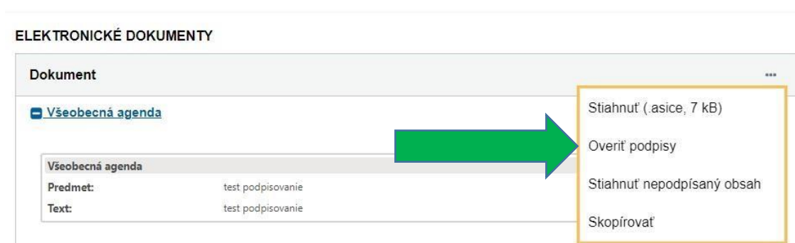
Obr. 7 – Overiť podpisy
