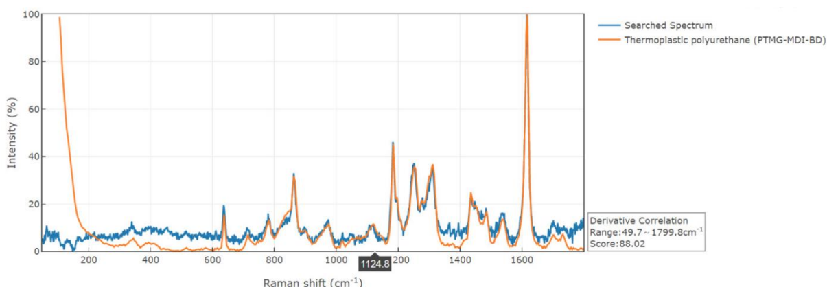
Obr. 3: Porovnanie nameraného Ramanového spektra s Ramanovým spektrom polyuretánu
